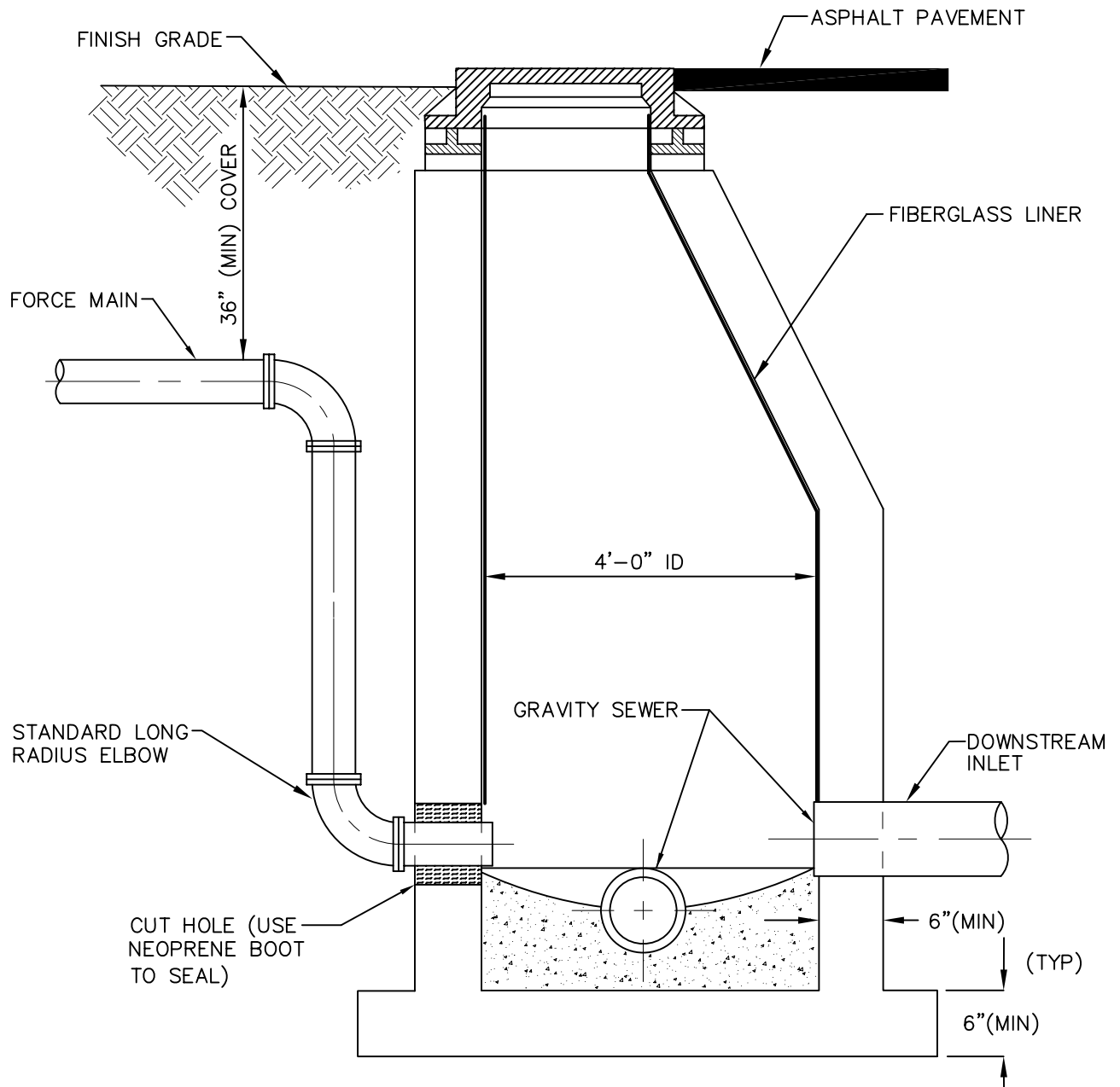
ELEVATION
